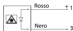
Collegamento cavo
