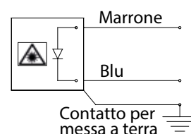
Collegamento cavo
