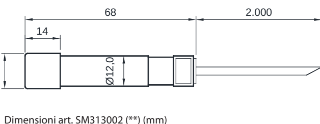
Dimensioni art. SM313002 (***) (mm)
