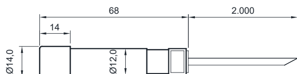
Dimensioni art. SM308010 (**) (mm)
