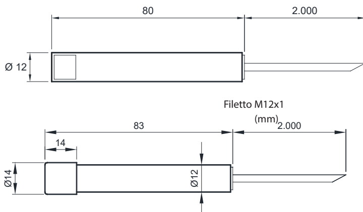
Dimensioni art. SM319017 e SM319018 (**) (mm)
